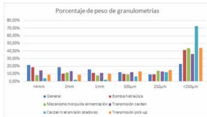
Figura2. Porcentaje del peso de los resultados de los 6 tamaños tamizados respecto el total de la muestra. Fuente: Ayudán C., 2021.
