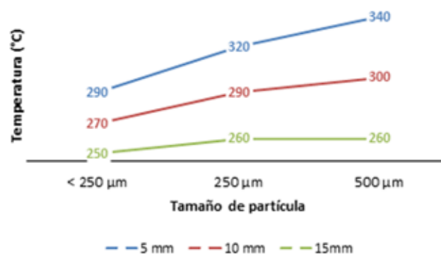
Figura3. Representación de la temperatura de ignición en función del tamaño de muestra para tres espesores de muestra (superior) y del espesor de la muestra para tres tamaños de partícula (inferior). Fuente: Val Agasca et al. (2019).
